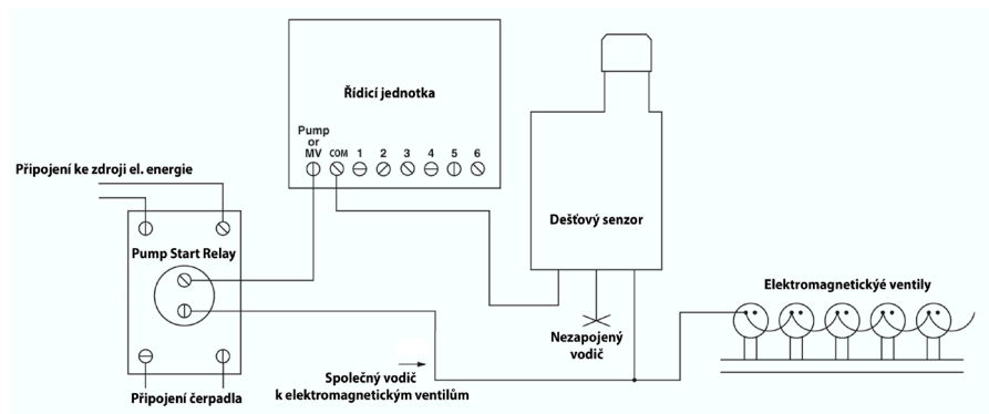
Obr. 4: Zapojení do řídicí jednotky bez svorek pro senzor, s ovládáním čerpadla
