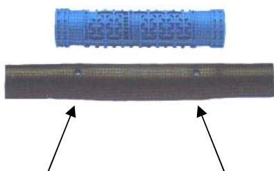
Zdvojený výtok vody z jednoho kapkovače TANDEM-GDF
